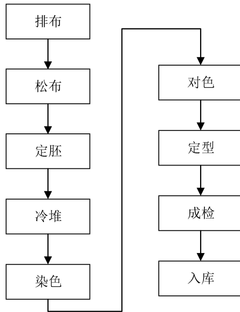
图 3.1.4 涤棉布生产工艺流程图
